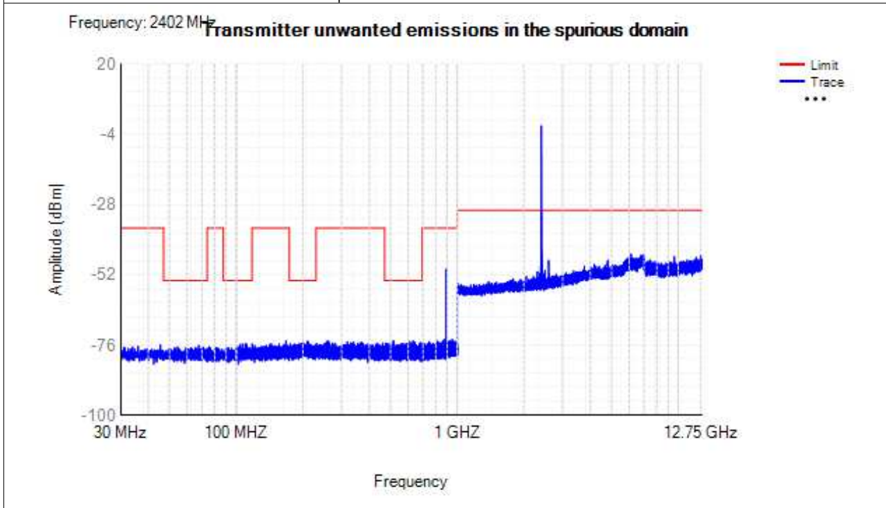
Tx. Spurious NVNT BLE 2M 2402MHz Ant1
