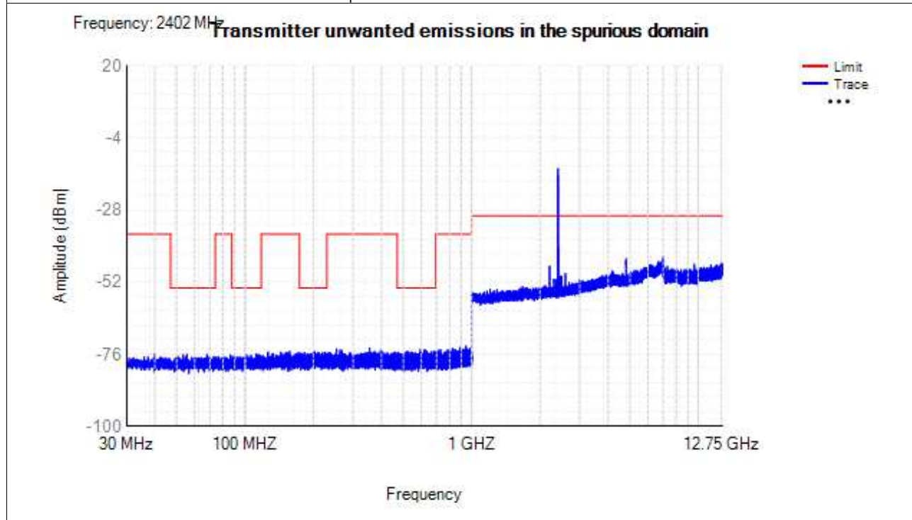
Tx. Spurious NVNT BLE 2M 2402MHz Ant1
