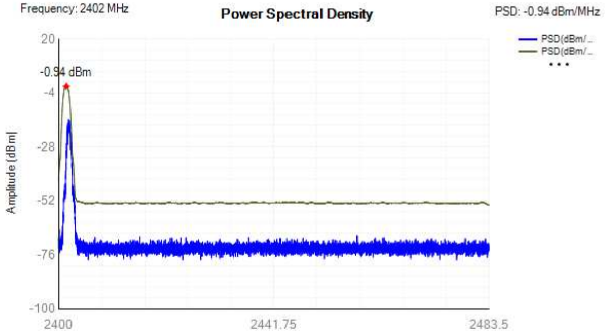
PSD NVNT BLE 1M 2402MHz Ant1
