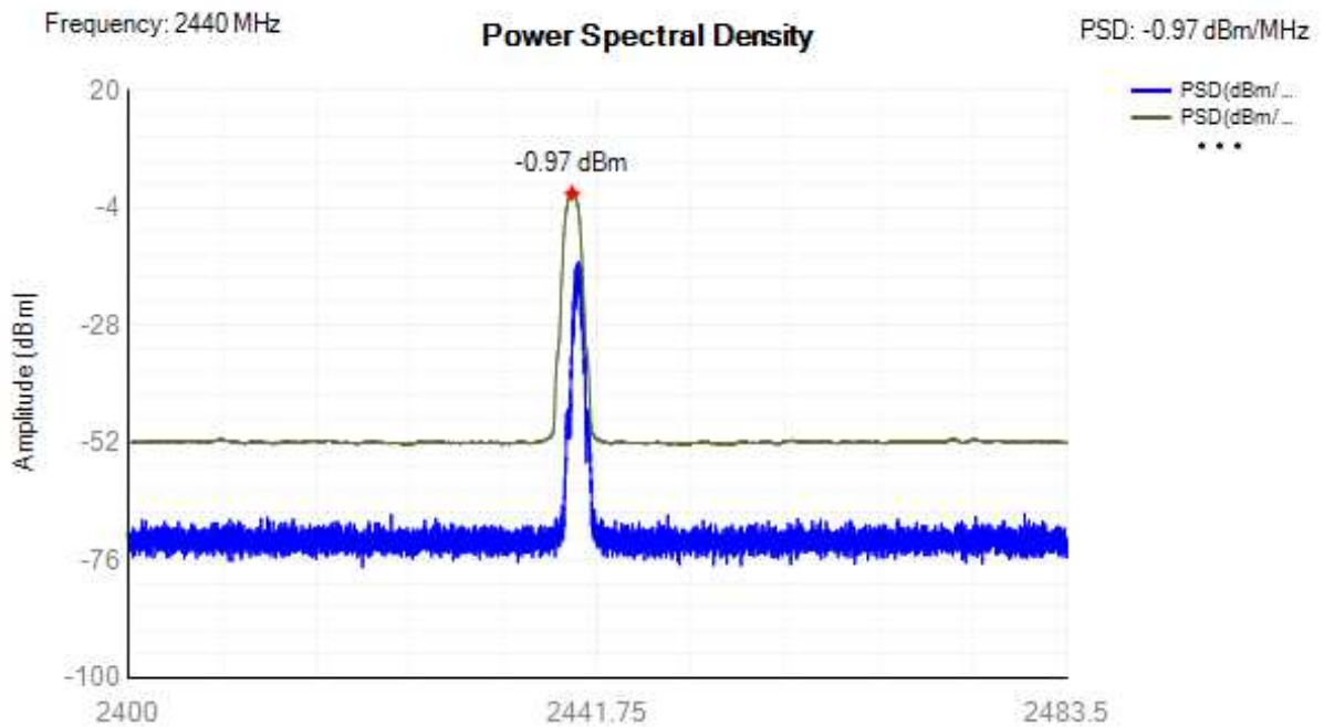
PSD NVNT BLE 1M 2440MHz Ant1
