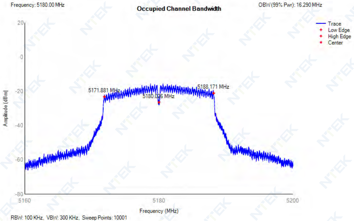
OBW NVNT 802.11ac20 5180MHz
