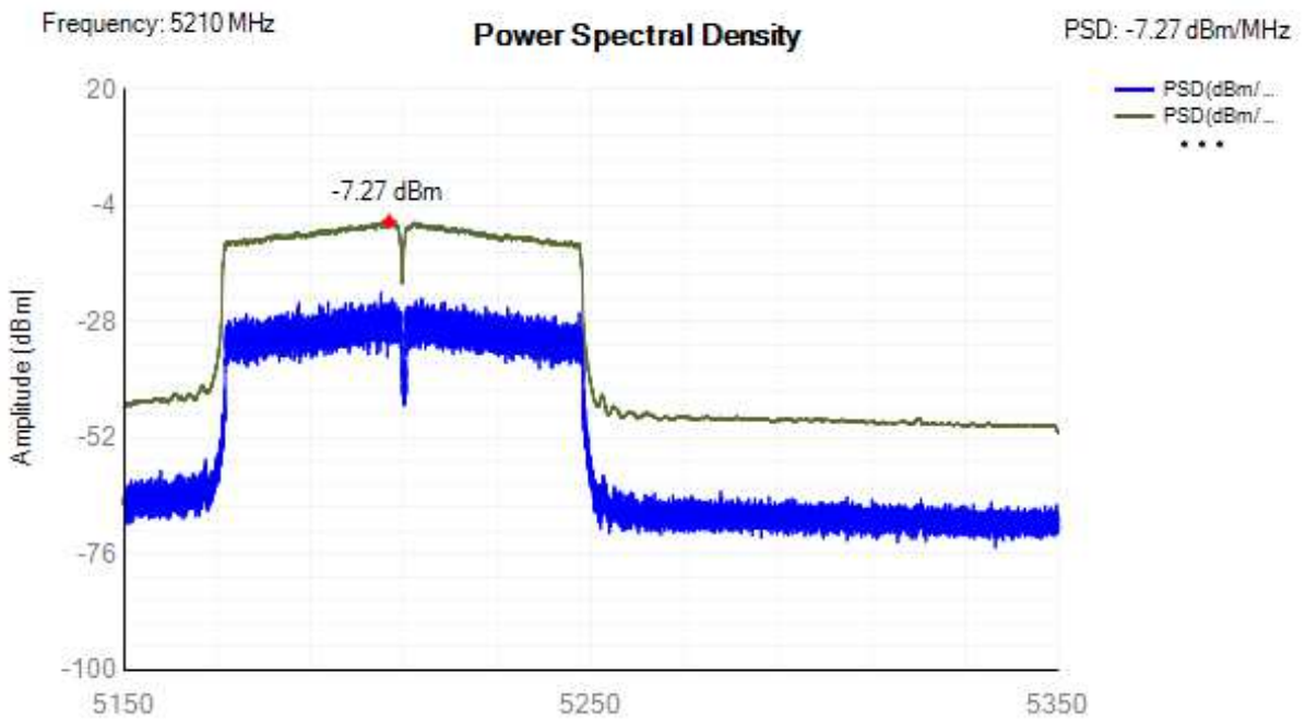
PSD NVNT ac80 5210MHz Ant1
