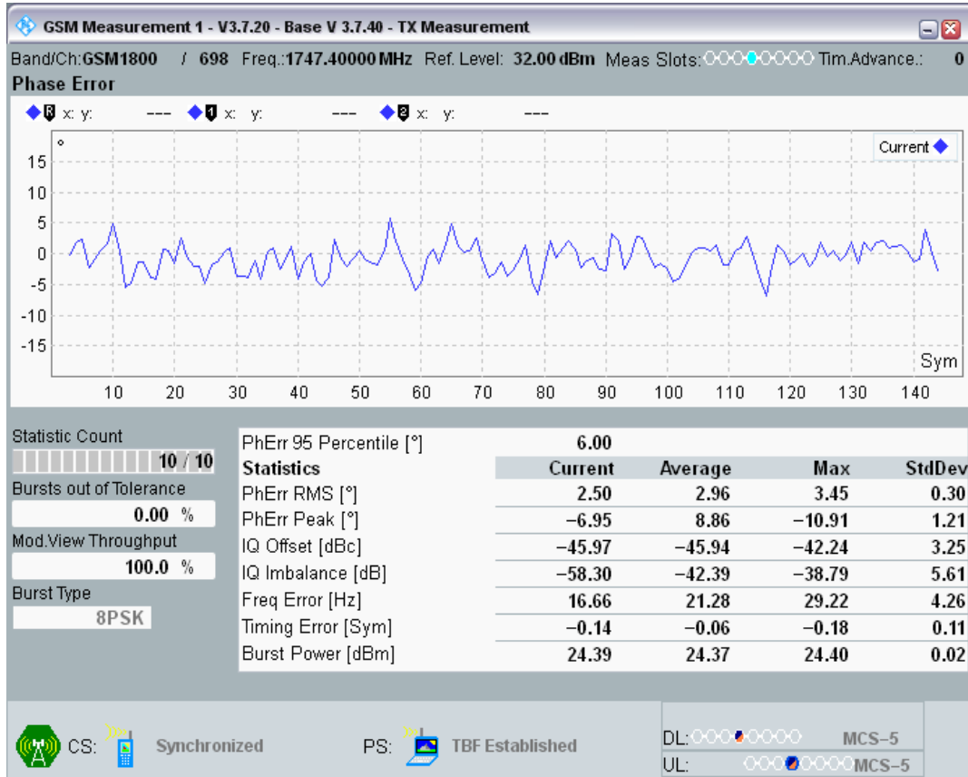
EGPRS1800 Channel=698 Gamma=5;5;5;5 RA250 @Sens1
