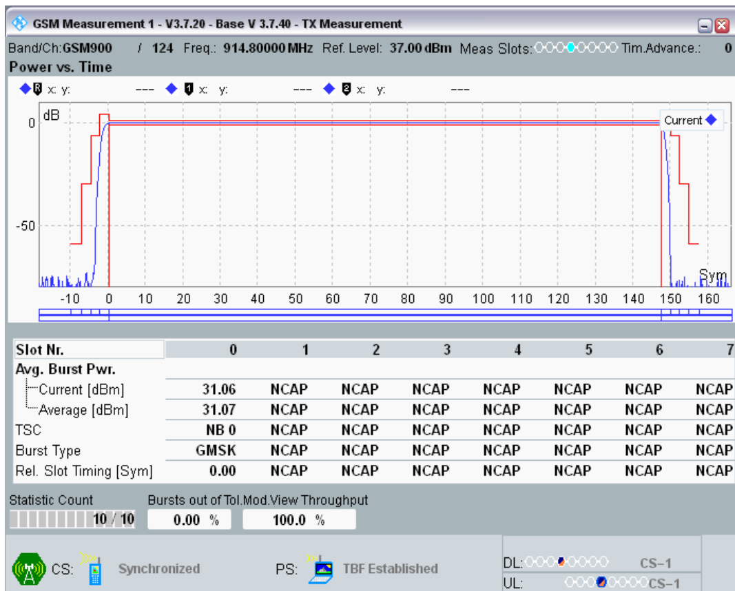
GPRS900 Channel=124 Gamma=5;5;5;5
