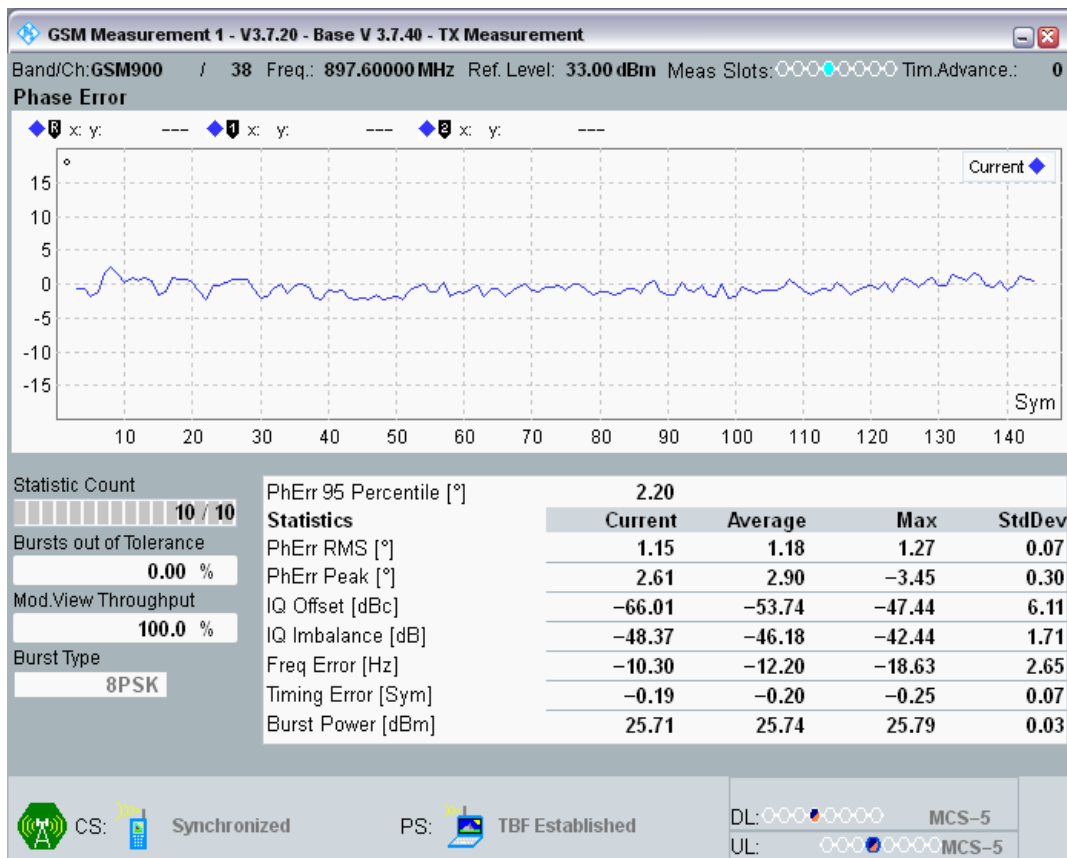
EGPRS900 Channel=38 Gamma=6;6;6;6 TU3 @1
