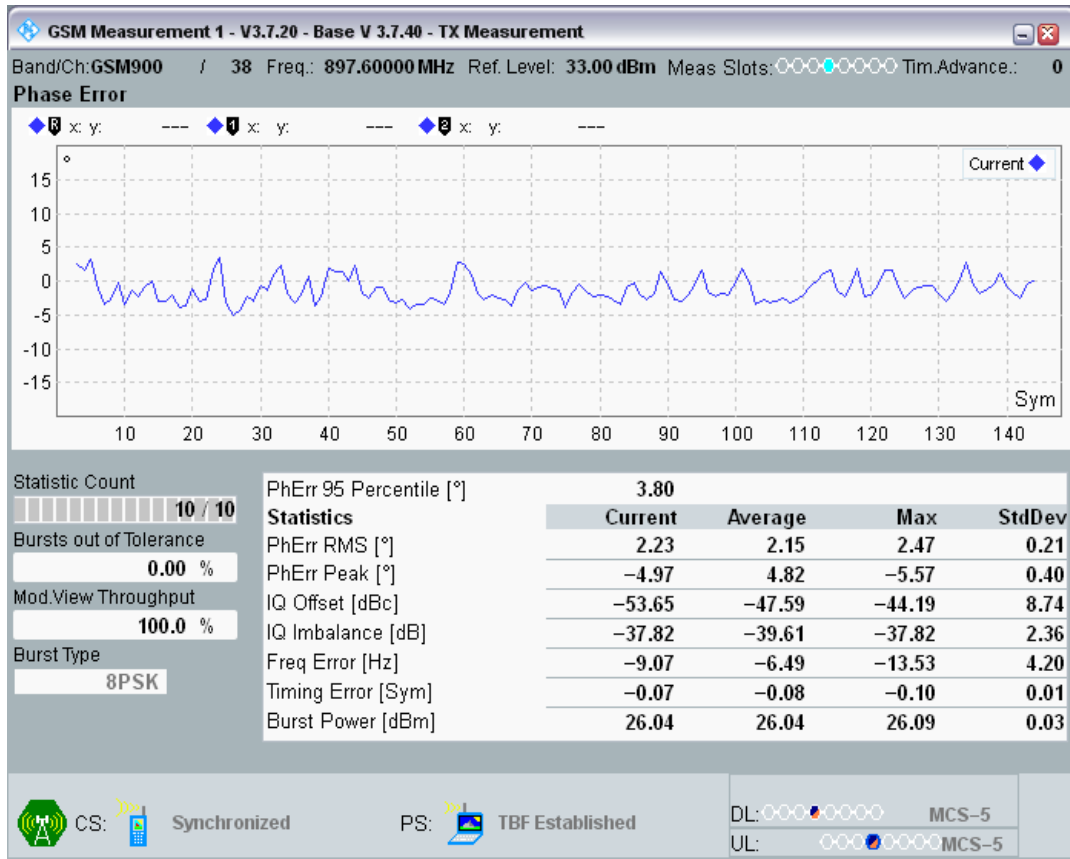
EGPRS900 Channel=38 Gamma=6;6;6 TU3 @19
