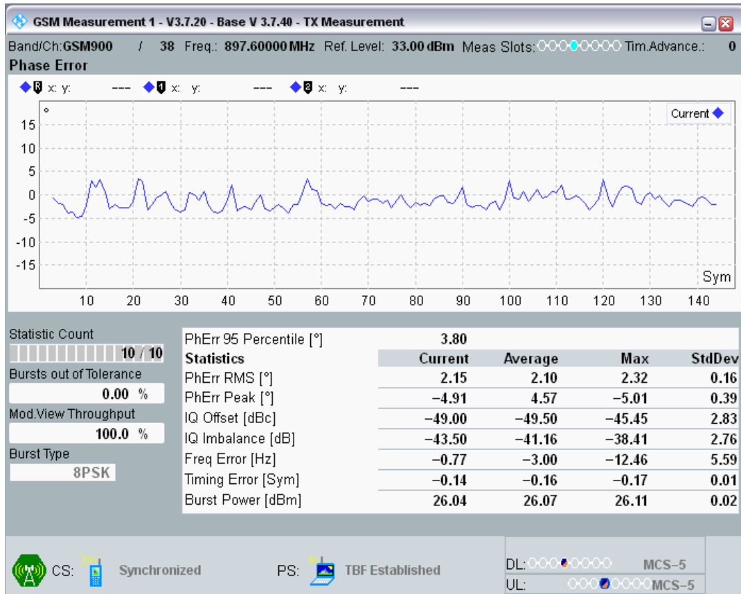
EGPRS900 Channel=38 Gamma=6;6;6 TU3 @19
