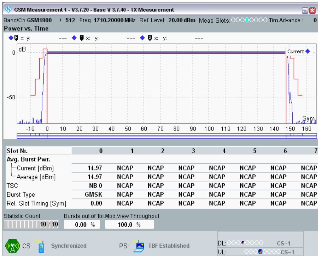
GPRS1800 Channel=512 Gamma=12;12;12;12
