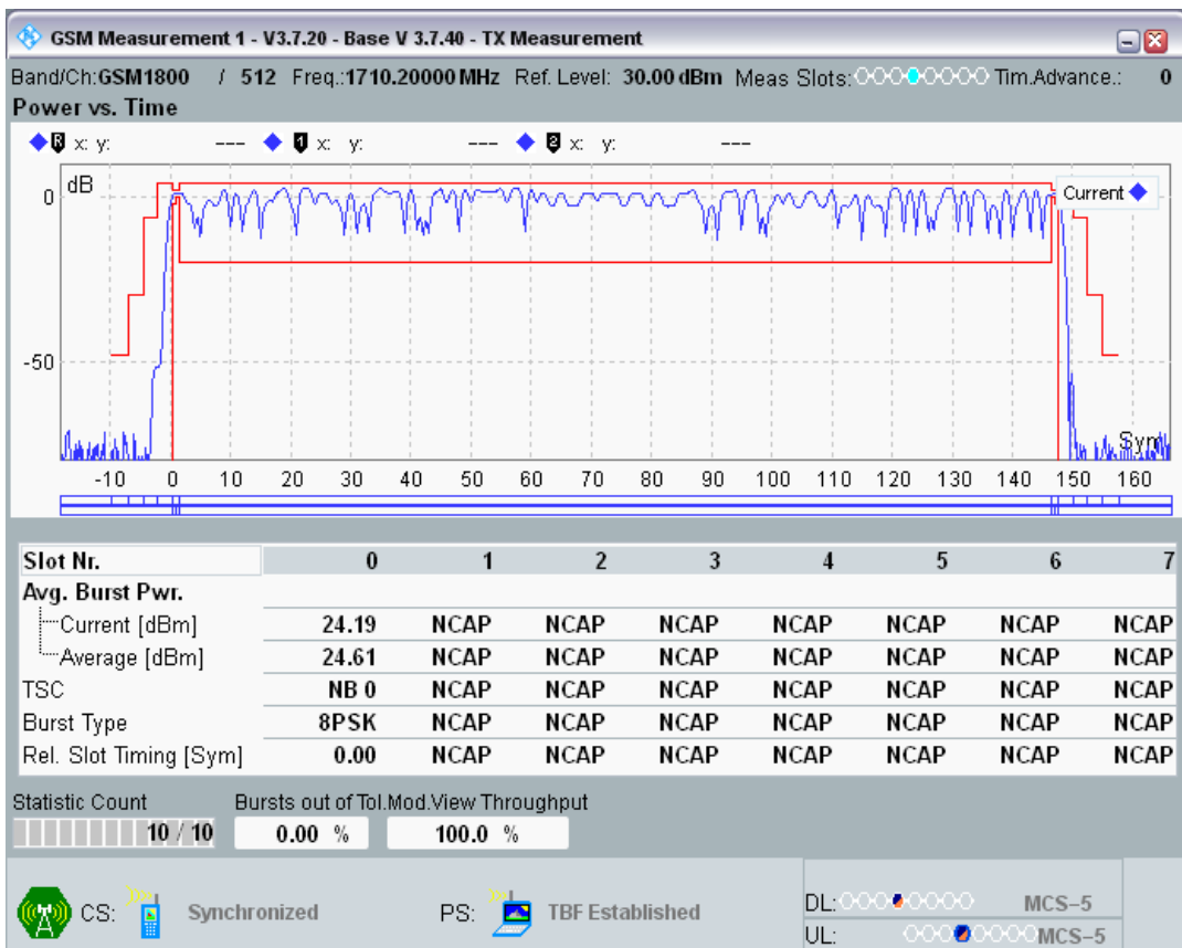
EGPRS1800 Channel=512 Gamma=8;8;8
