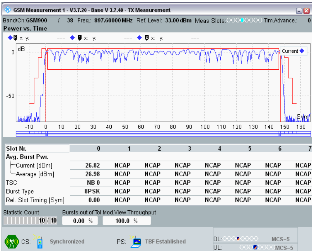
EGPRS900 Channel=38 Gamma=8;8;8;8
