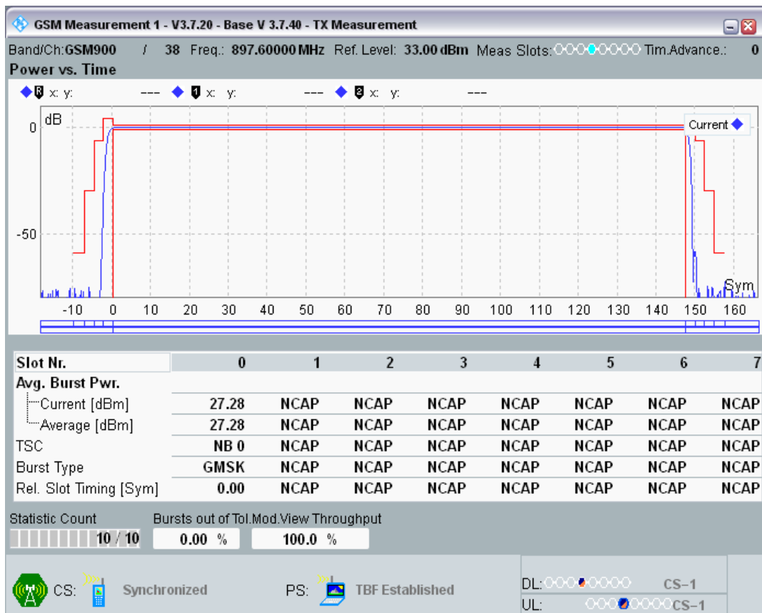
GPRS900 Channel=38 Gamma=5;5;5
