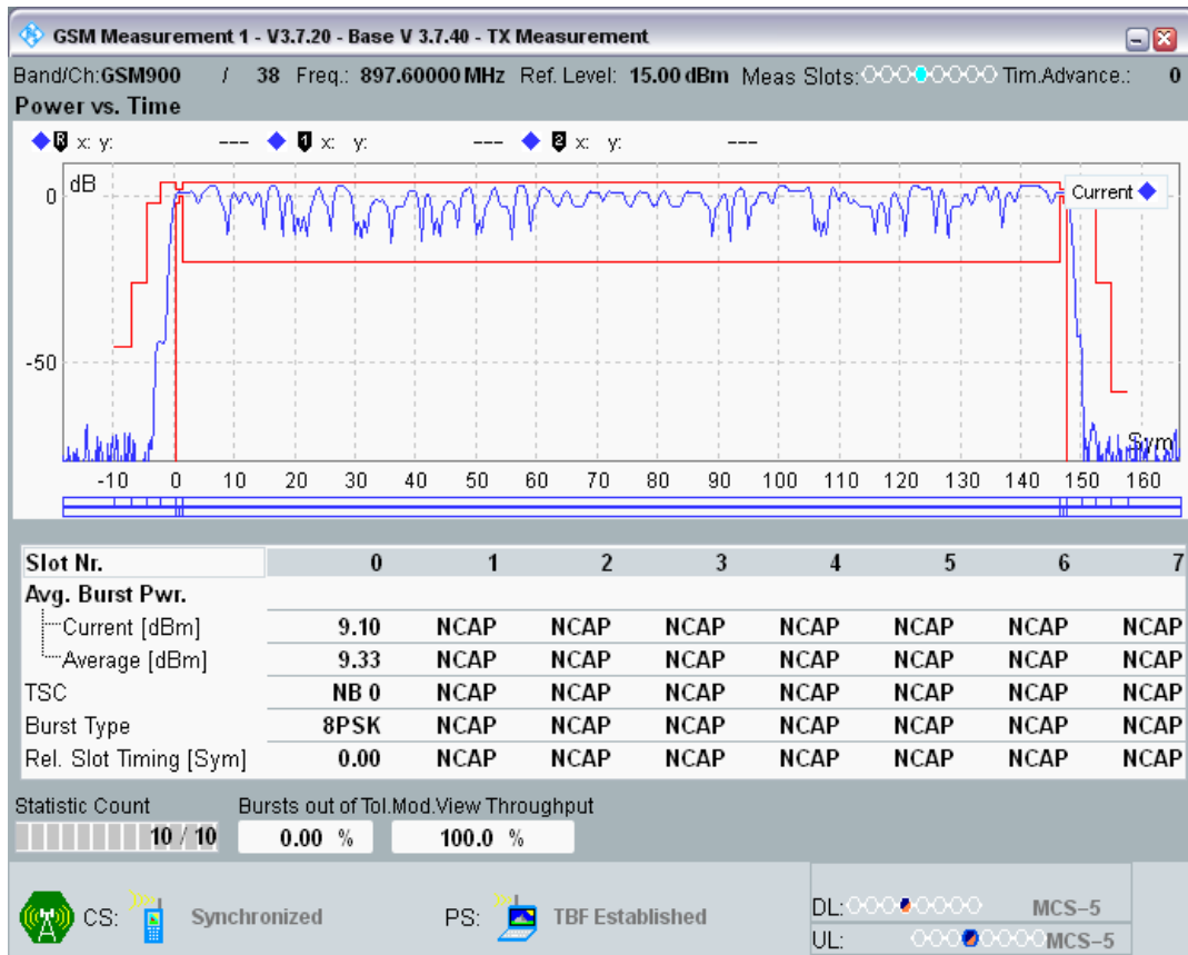
EGPRS900 Channel=38 Gamma=16;16;16;16
