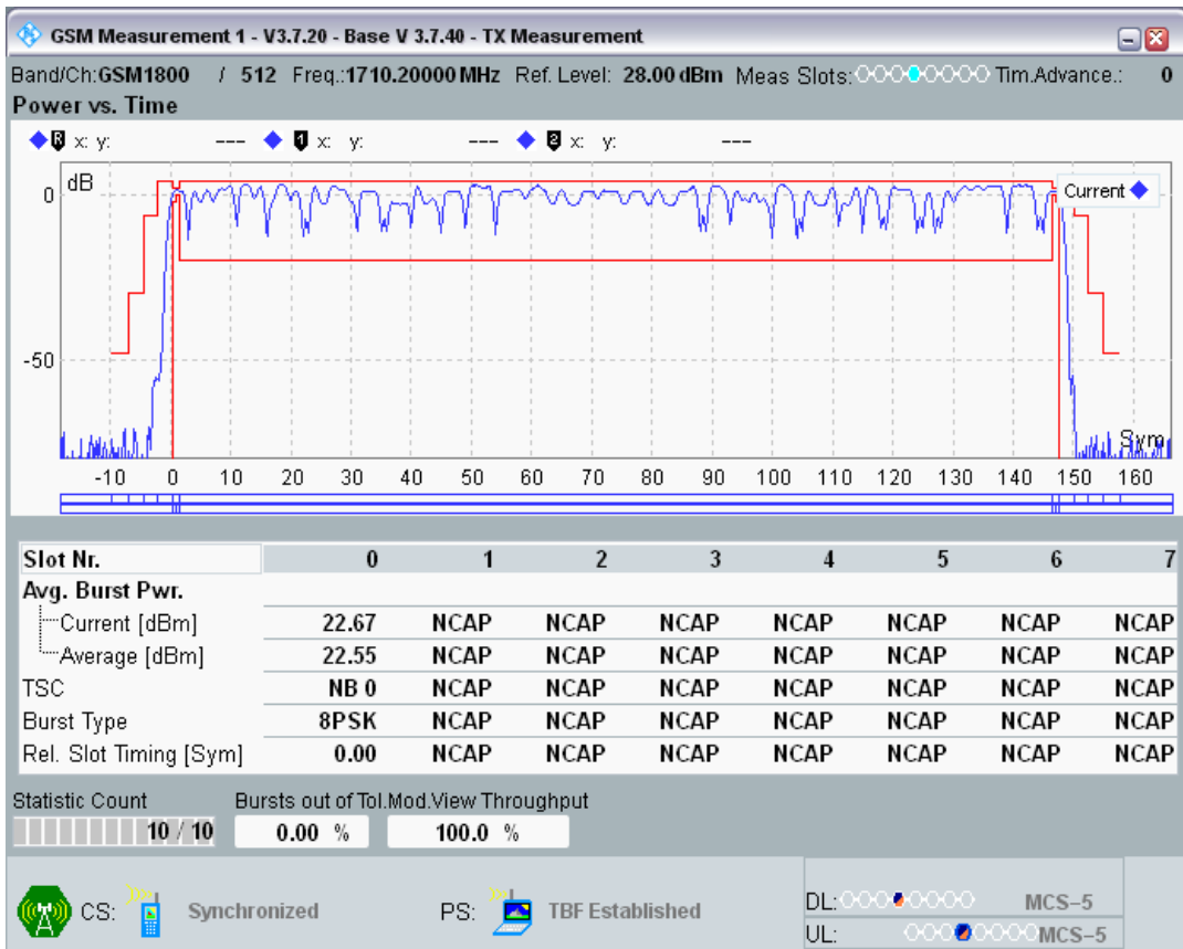
EGPRS1800 Channel=512 Gamma=6;6;6
