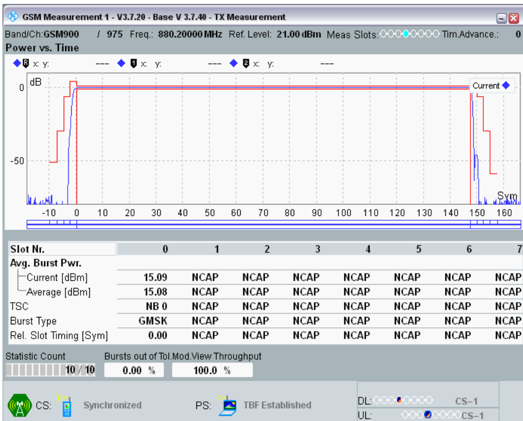
GPRS900 Channel=975 Gamma=13;13;13;13
