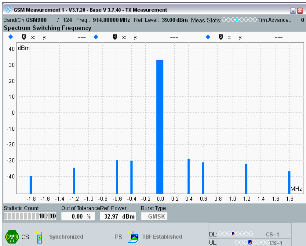
GPRS900 Channel=124 Gamma=3;3;3
