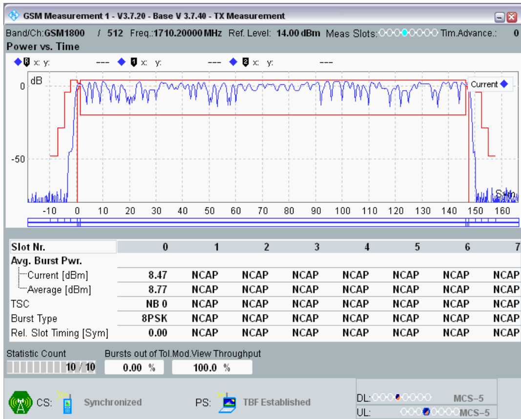
EGPRS1800 Channel=512 Gamma=15;15;15;15
