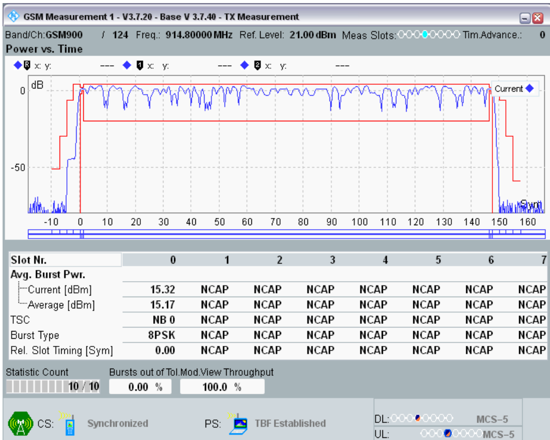
EGPRS900 Channel=124 Gamma=13;13;13;13
