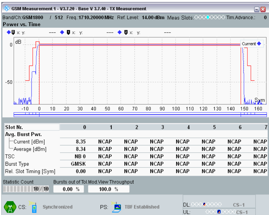
GPRS1800 Channel=512 Gamma=15;15;15;15
