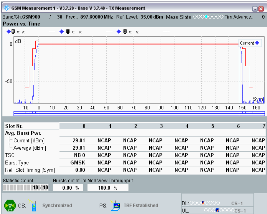
GPRS900 Channel=38 Gamma=6;6;6;6
