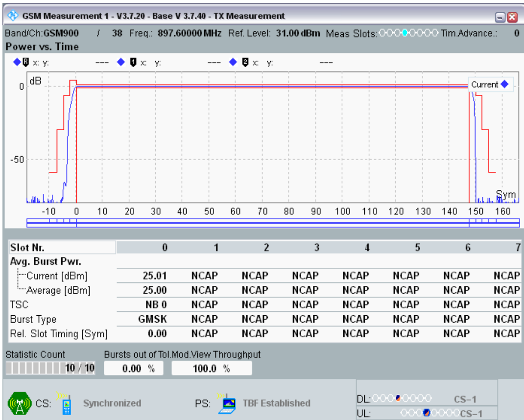
GPRS900 Channel=38 Gamma=9;9;9
