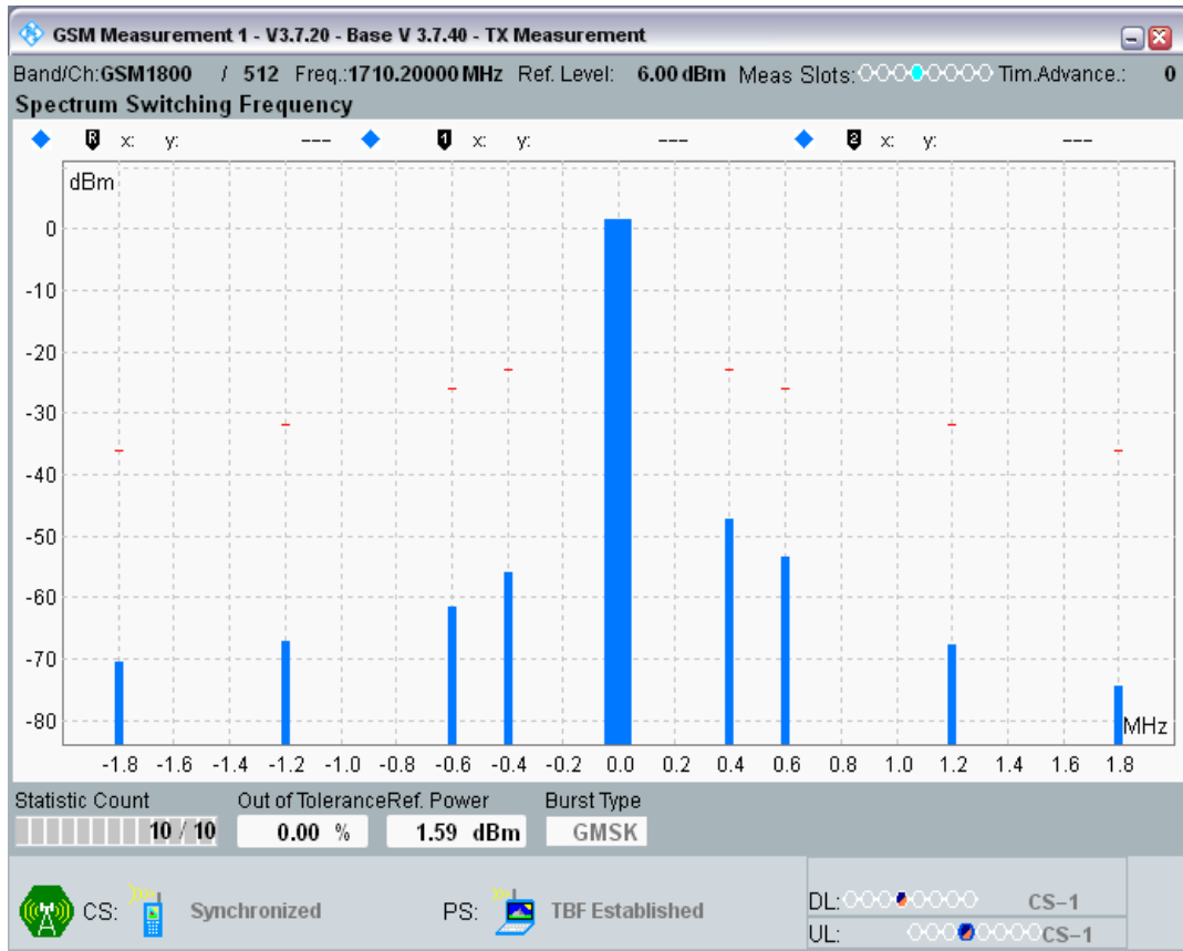
GPRS1800 Channel=512 Gamma=3;3;3
