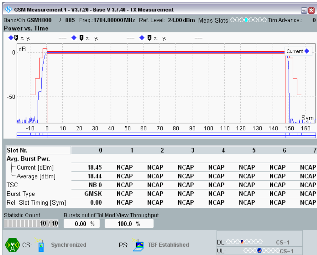
GPRS1800 Channel=885 Gamma=10;10;10;10
