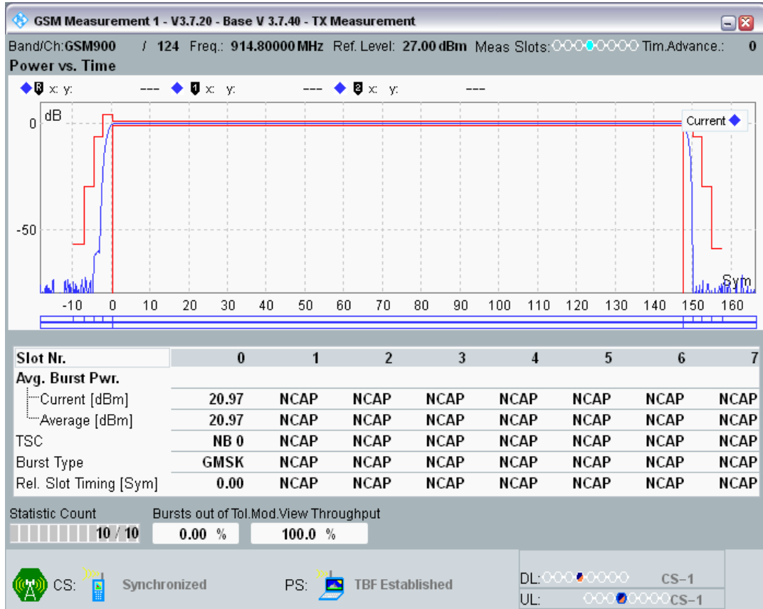
GPRS900 Channel=124 Gamma=10;10;10;10
