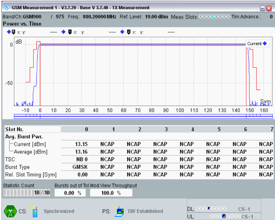
GPRS900 Channel=975 Gamma=14;14;14;14
