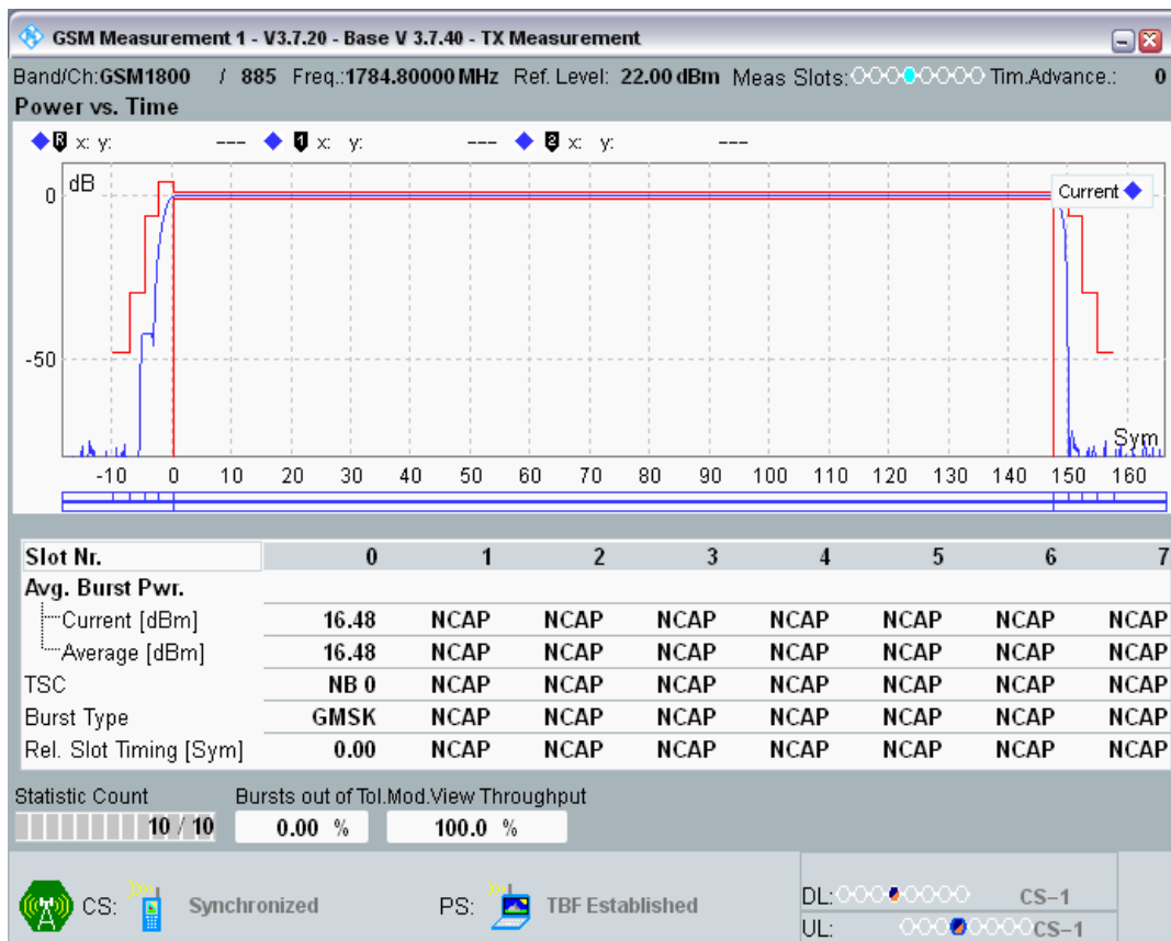
GPRS1800 Channel=885 Gamma=11;11;11;11
