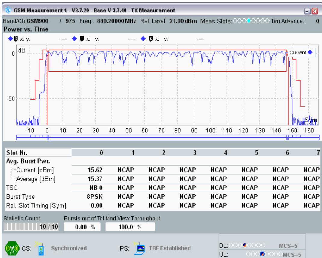
EGPRS900 Channel=975 Gamma=13;13;13;13
