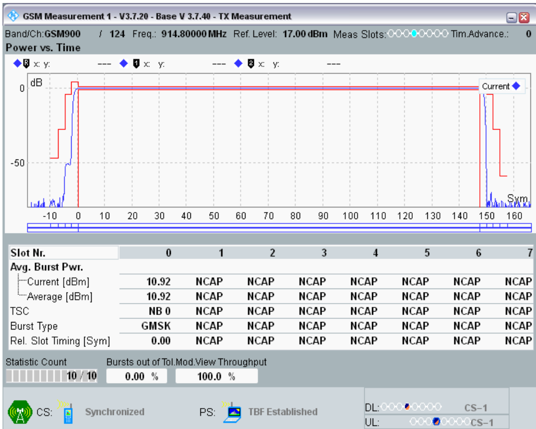
GPRS900 Channel=124 Gamma=15;15;15;15
