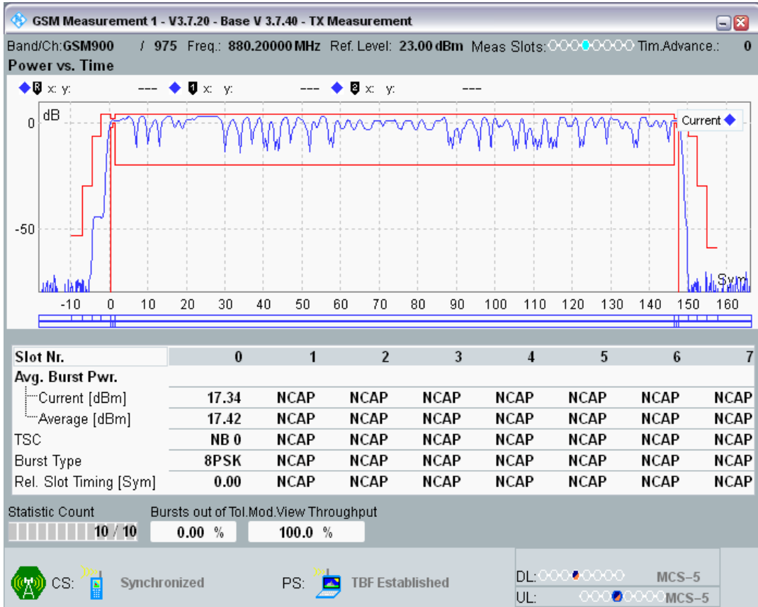
EGPRS900 Channel=975 Gamma=12;12;12;12
