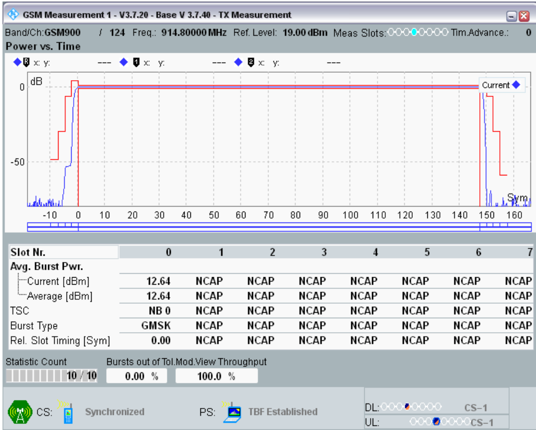
GPRS900 Channel=124 Gamma=14;14;14;14
