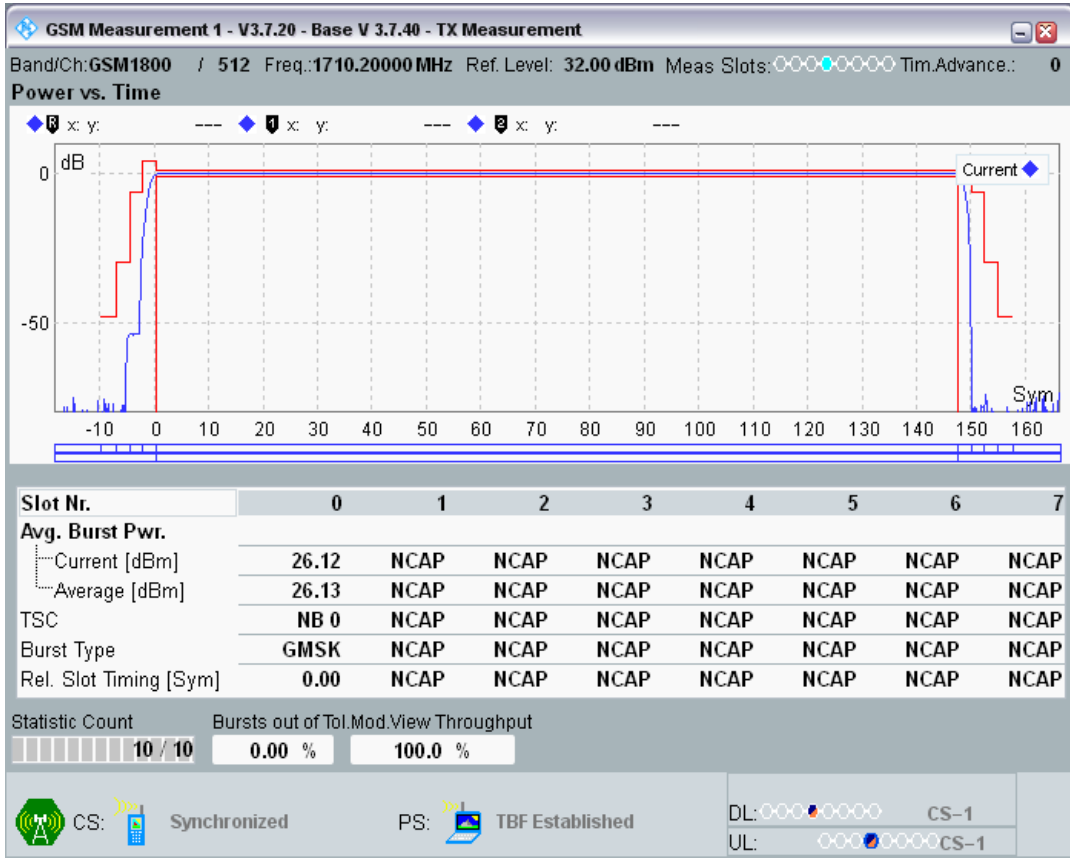
GPRS1800 Channel=512 Gamma=6;6;6
