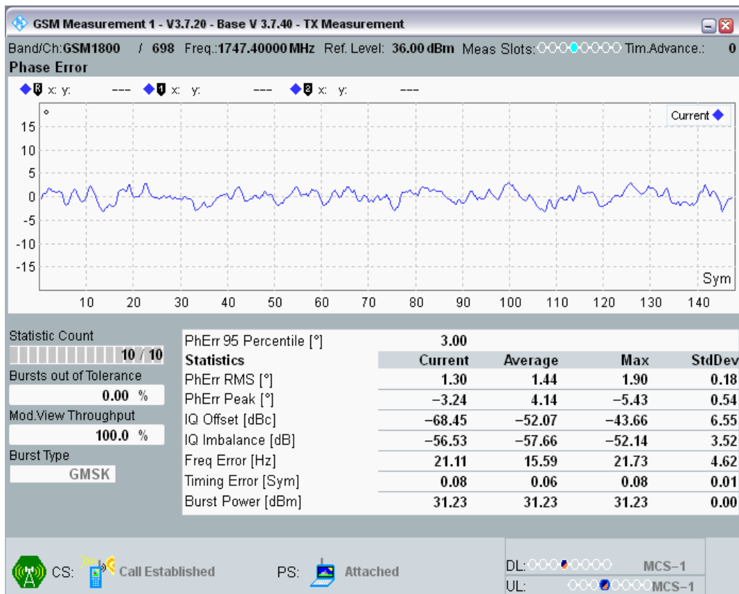
GSM1800 Channel=698 PCL=0 TU50 @Sens1
