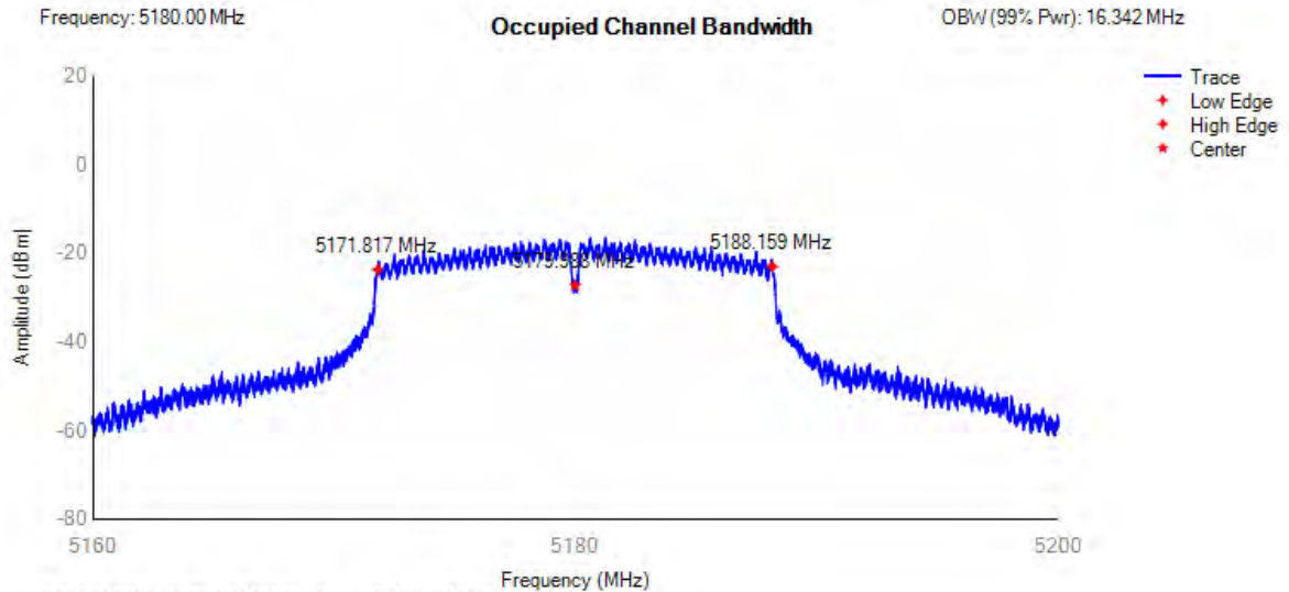
OBW NVNT 802.11a 5180MHz
