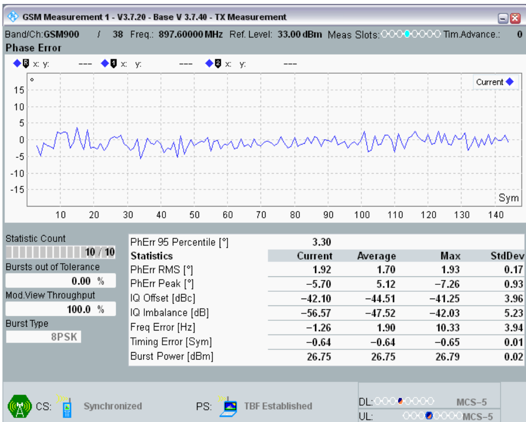
EGPRS900 Channel=38 Gamma=6;6;6;6 TU3 @5
