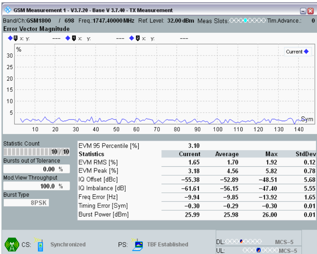
EGPRS1800 Channel=698 Gamma=5;5;5;5 TU3 @2
