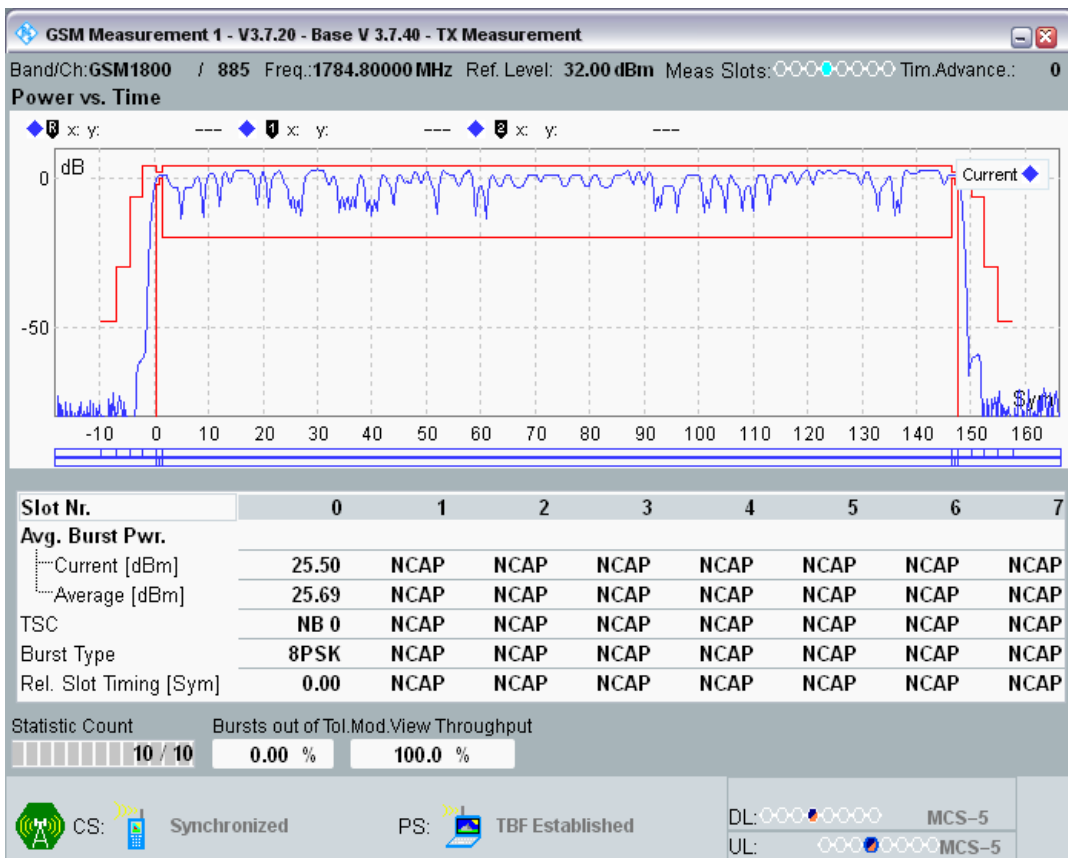
EGPRS1800 Channel=885 Gamma=6;6;6;6
