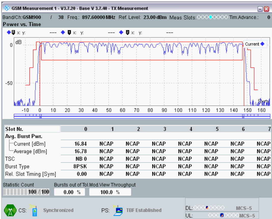
EGPRS900 Channel=38 Gamma=12;12;12;12
