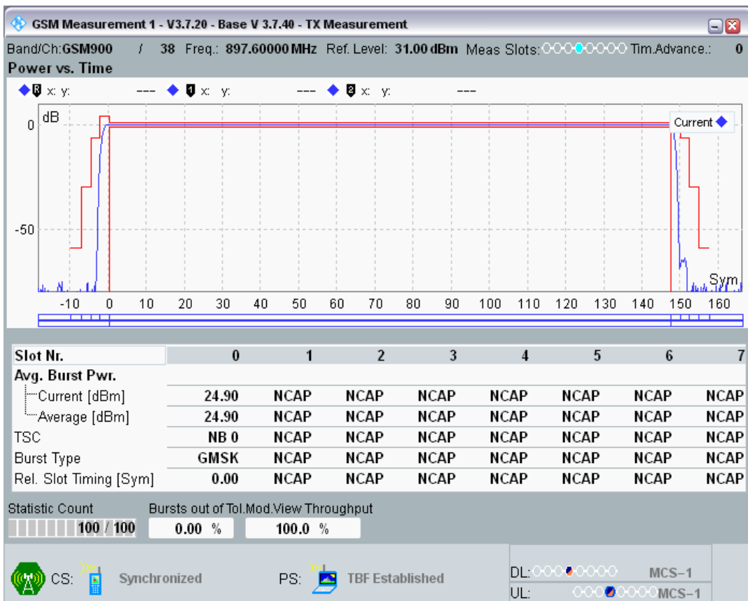
GPRS900 Channel=38 Gamma=9;9;9
