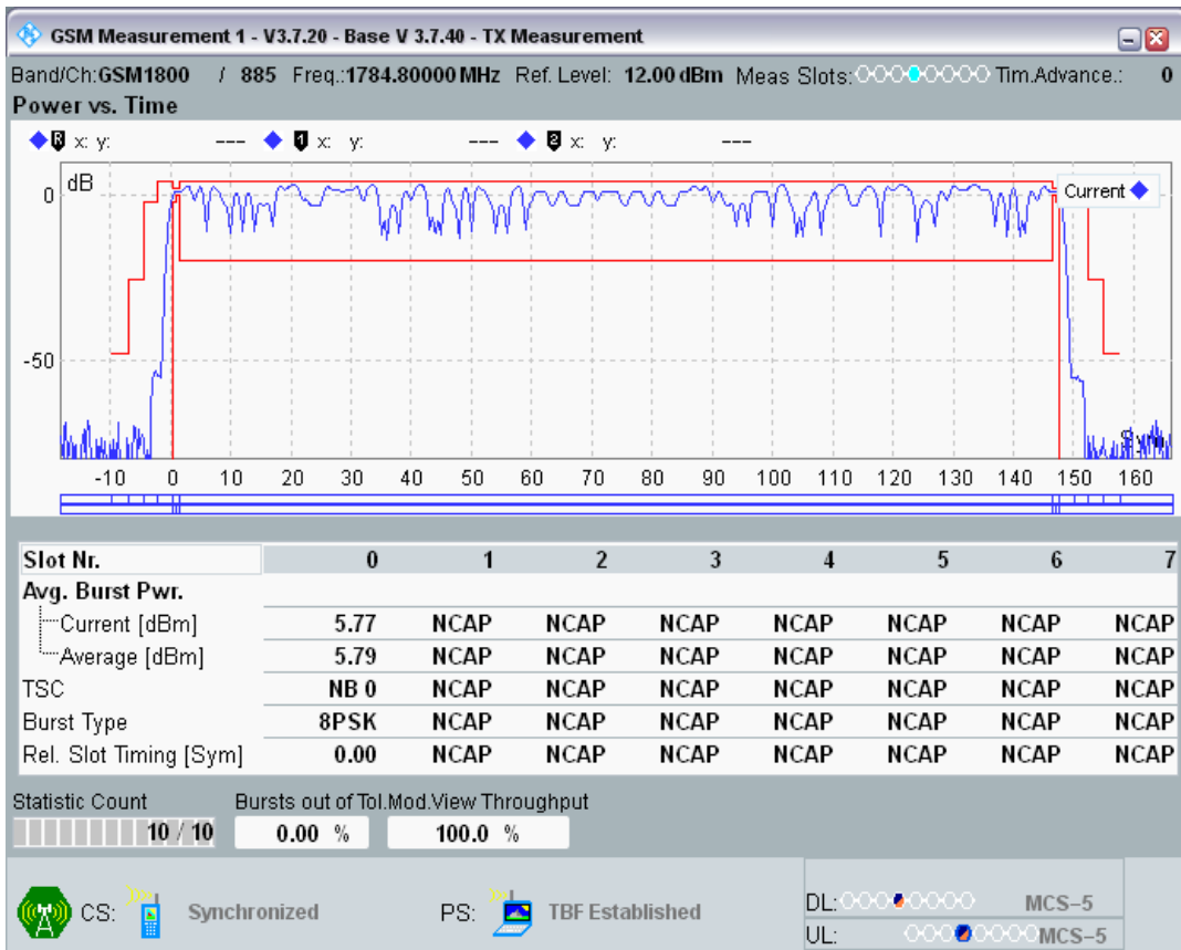
EGPRS1800 Channel=885 Gamma=14;14;14;14
