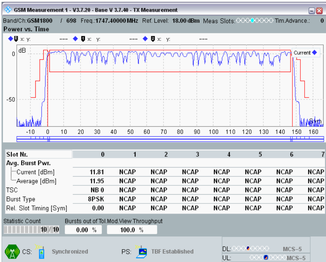
EGPRS1800 Channel=698 Gamma=13;13;13;13
