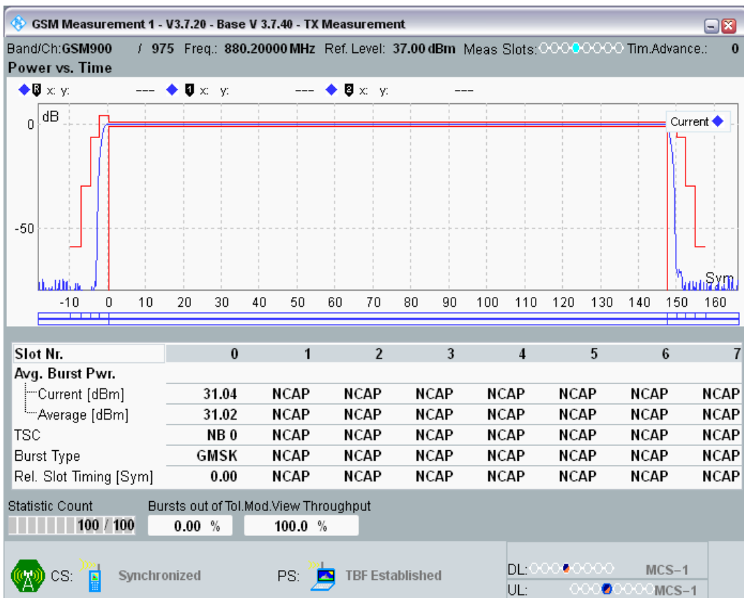
GPRS900 Channel=975 Gamma=5;5;5;5
