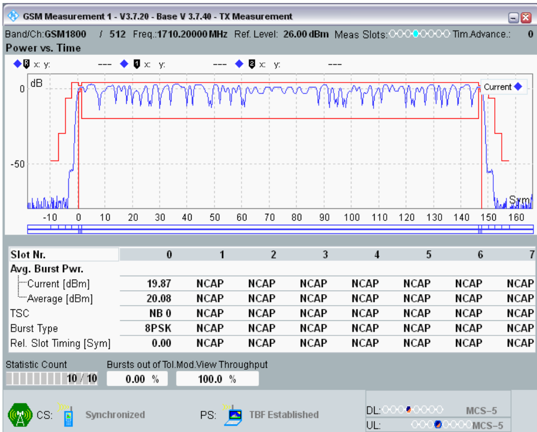
EGPRS1800 Channel=512 Gamma=9;9;9;9
