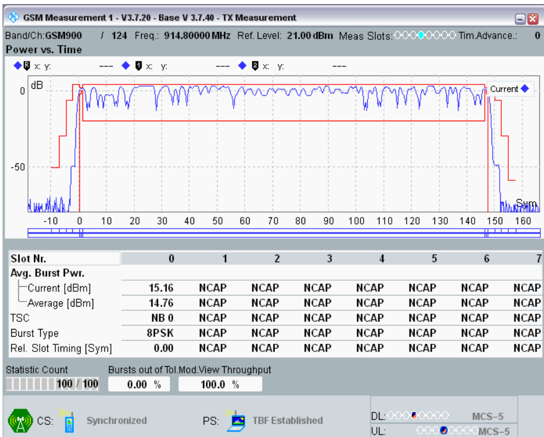
EGPRS900 Channel=124 Gamma=13;13;13;13
