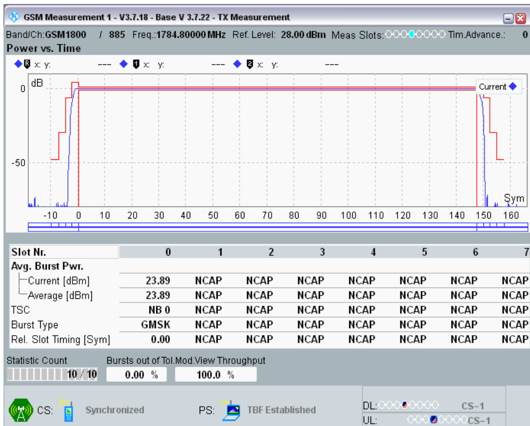
GPRS900 Channel=124 Gamma=12;12;12;12
