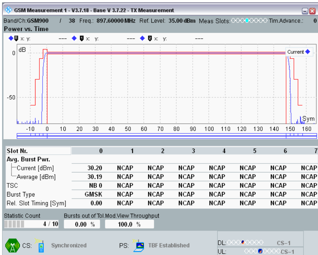
GPRS900 Channel=38 Gamma=8;8;8;8
