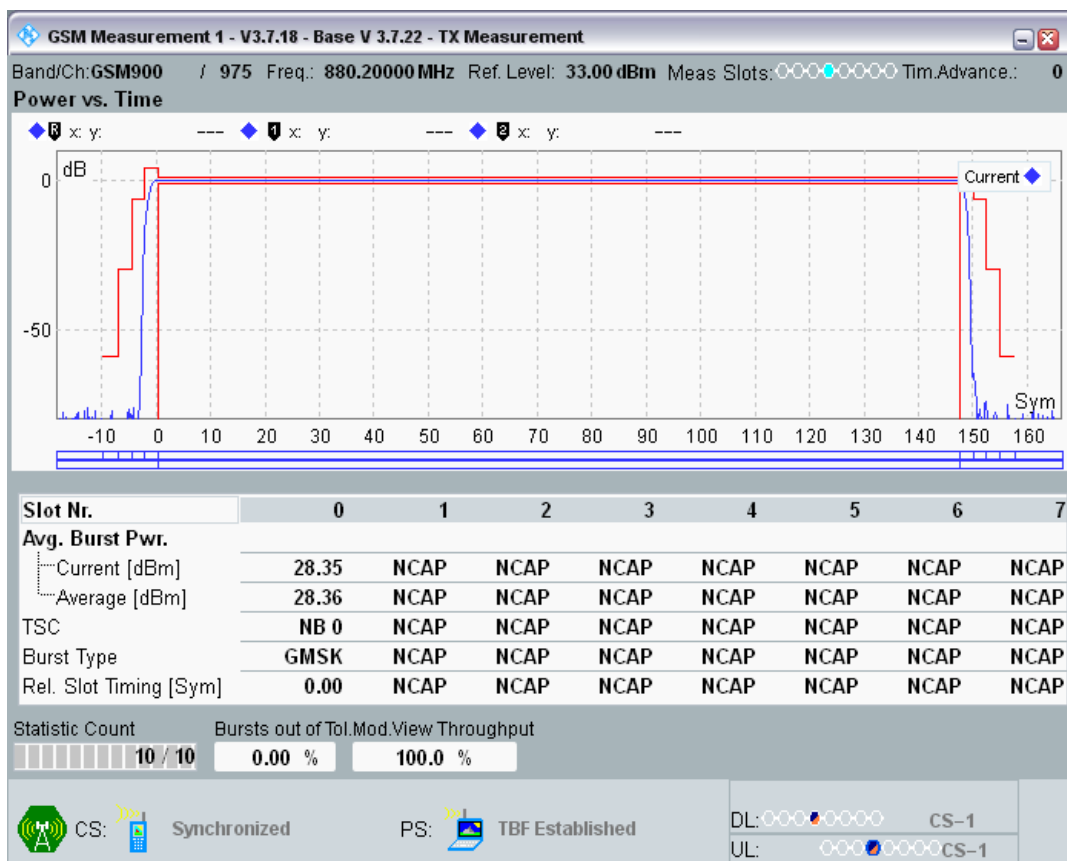
GPRS900 Channel=975 Gamma=9;9;9;9
