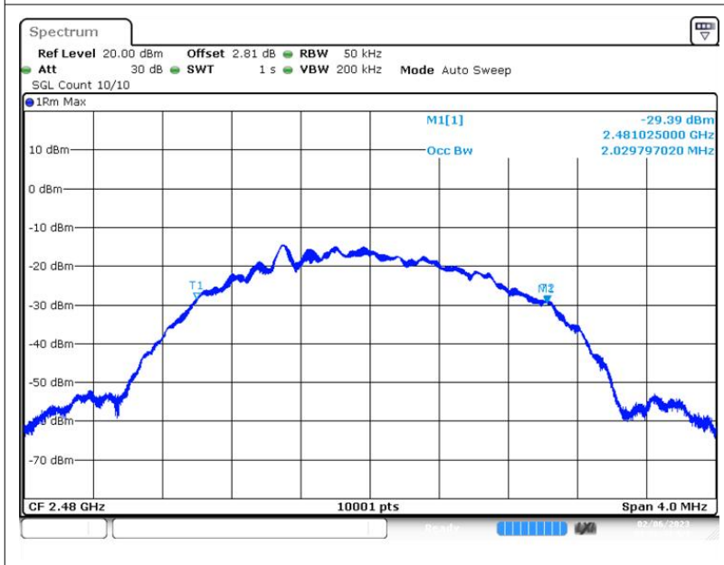
OBW NVNT BLE 2M 2480MHz Ant1
