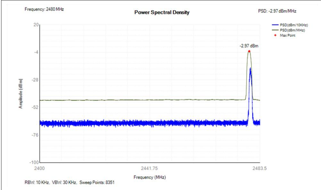
PSD NVNT BLE 2M 2402MHz Ant1
