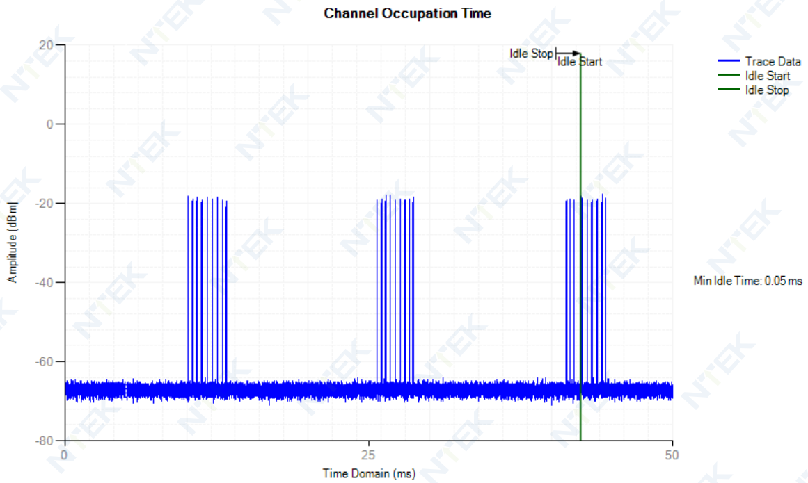
COT NVNT 802.11ac80 5210MHz
