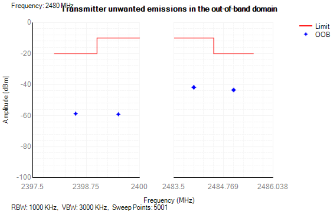
Tx. Emissions OOB NVNT BLE 1M 2480MHz Ant1
